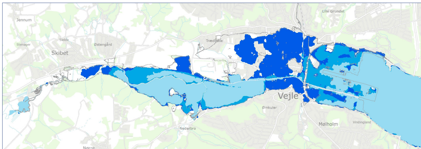
Figur 6: Oversvømmelsesudbredelse for en stormflod med den statistisk gentagelsesperiode på 100 år i 2019 (lyseblå, kote 1,62 m), 2065 (lyseblå samt mellemblå, kote 1,91 m) og 2115 (lyseblå, mellemblå og mørkeblå, kote 2,37 m).
